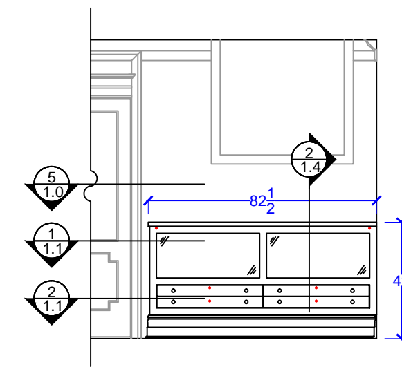
2 ELEVATION Scale: 1/4"=1'-0"
