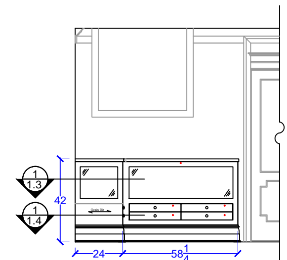
4 ELEVATION Scale: 1/4"=1'-0"
