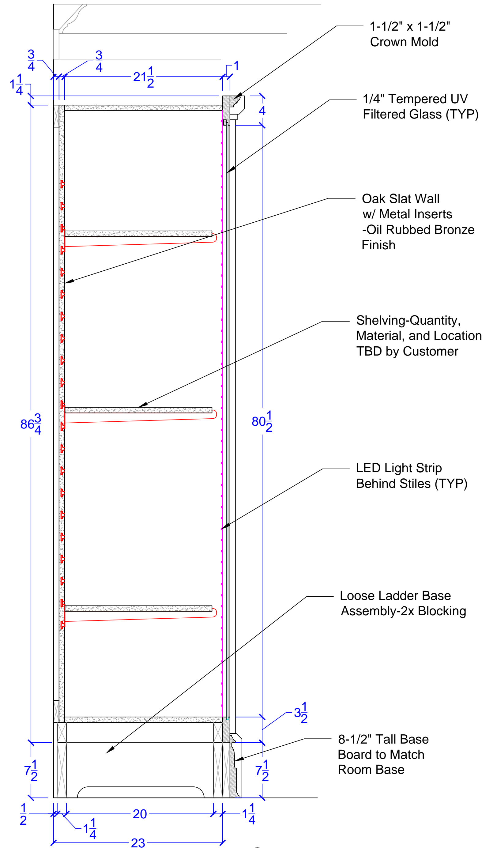
2 SECTION 1.3 SCALE: 1-1/2"=1'-0"
